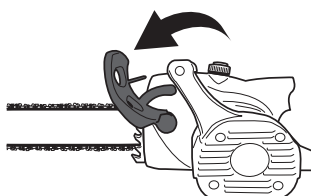
Fig. 17 Poignée de frein [2] enclenchée: la scie s'arrête dès que le frein est enclenché (Fig. 17).
